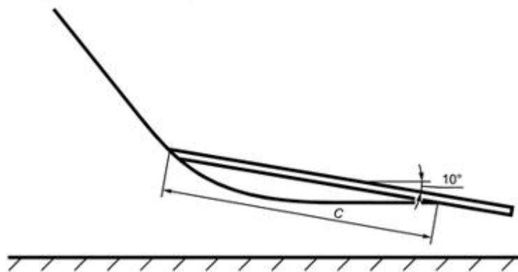
Рисунок 5 – Конечный участок горки типа 1
