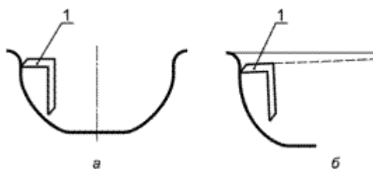
Верхняя плоскость шаблона горизонтальна. Профиль соответствует заданным требованиям.
