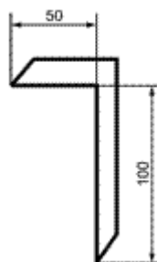
Рисунок А.3 – Шаблон для измерения профиля горки
