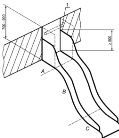
Рисунок 2 – Бортики и защитная перекладина пристраиваемой горки
